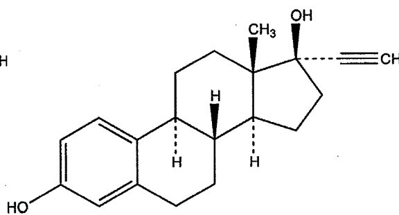
Ethinyl Estradiol C 20 H 24 O 2 M.W. 296.40
