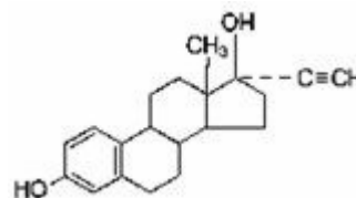
Ethinyl estradiol
