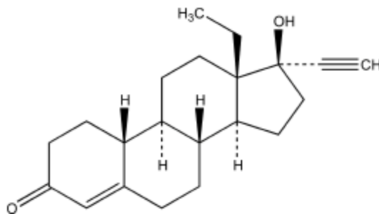
Norgestrel M.W. 312.45
