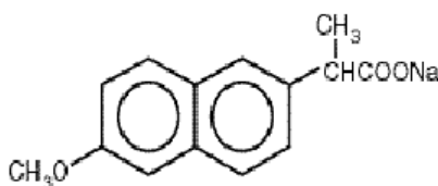
Naproxen sodium
