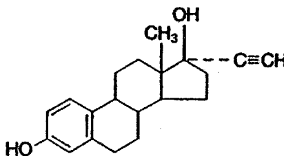
ETHINYL ESTRADIOL
