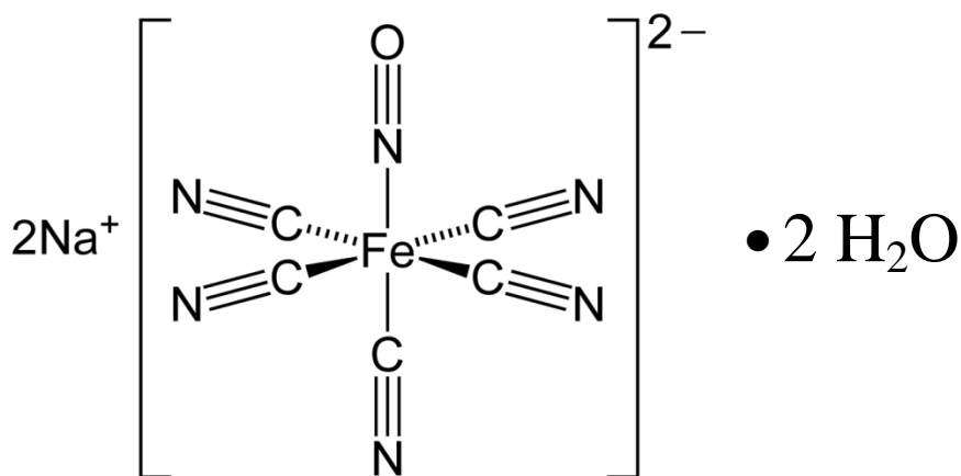
Sodium Nitroprusside
